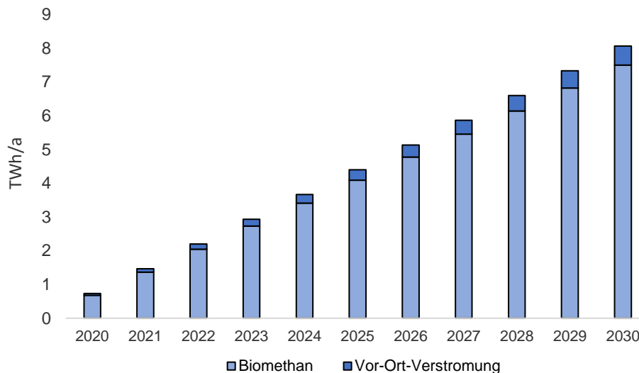
Abbildung 2: Zusätzlicher Ausbau von Biogas (kumuliert) bis 2030
